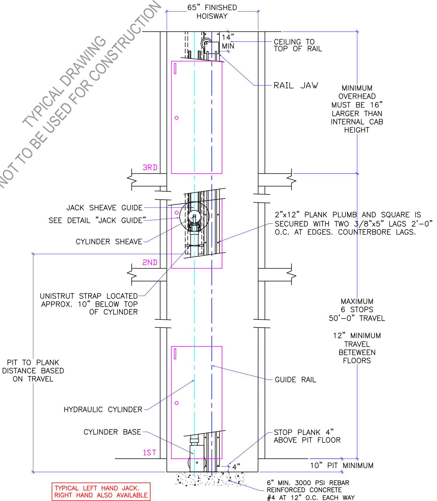
VIEW A-A
